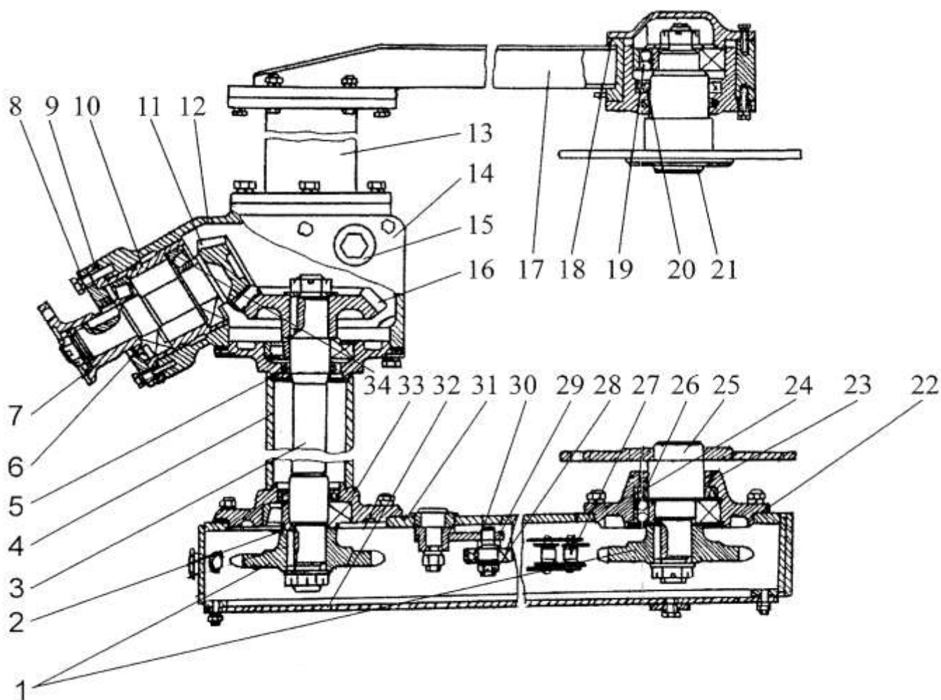
Рисунок 2 – Привод щетки
