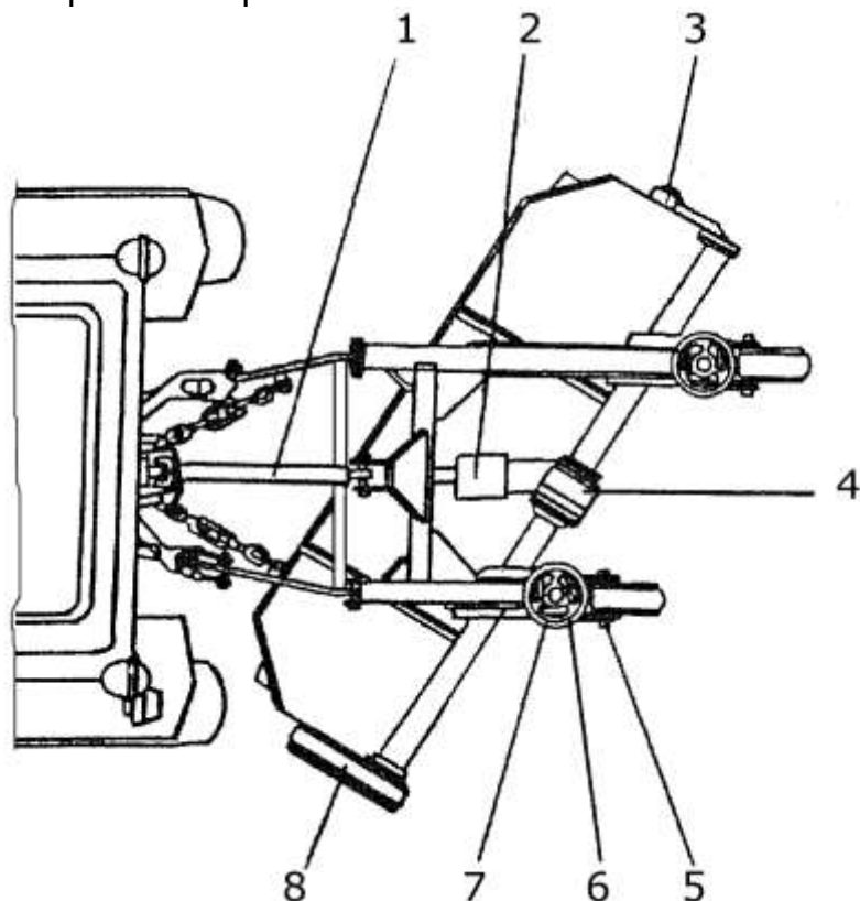
Рисунок 6 – Схема смазки
